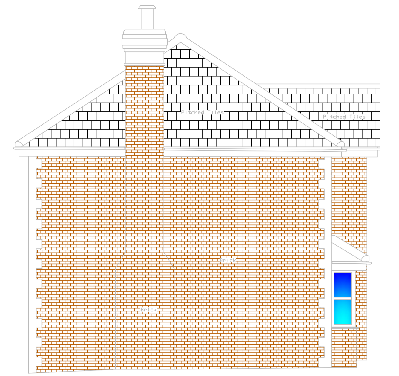
ELEVATION 2
