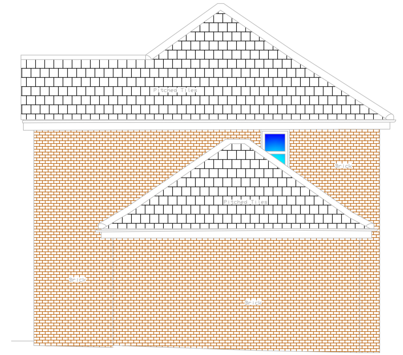
ELEVATION 4
