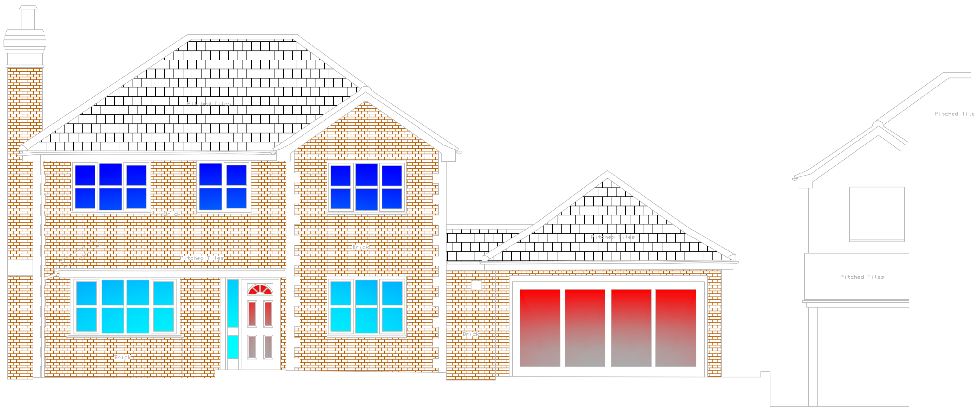
ELEVATION 1
